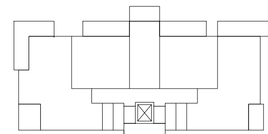
SCHEMAT - 3 PIETRO
